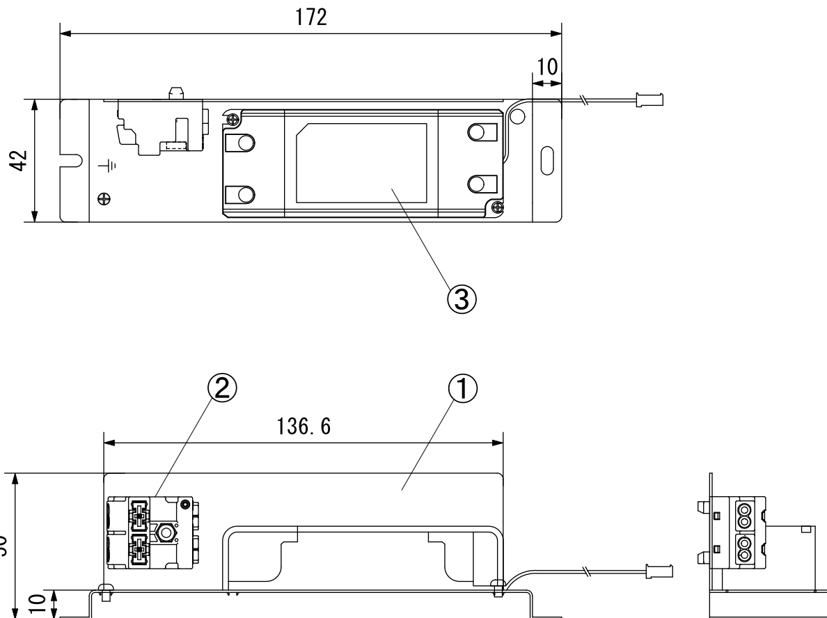
UDL-1161**, UDL-1162**, UDL-1163**, UDL-1904**専用電源ユニット
