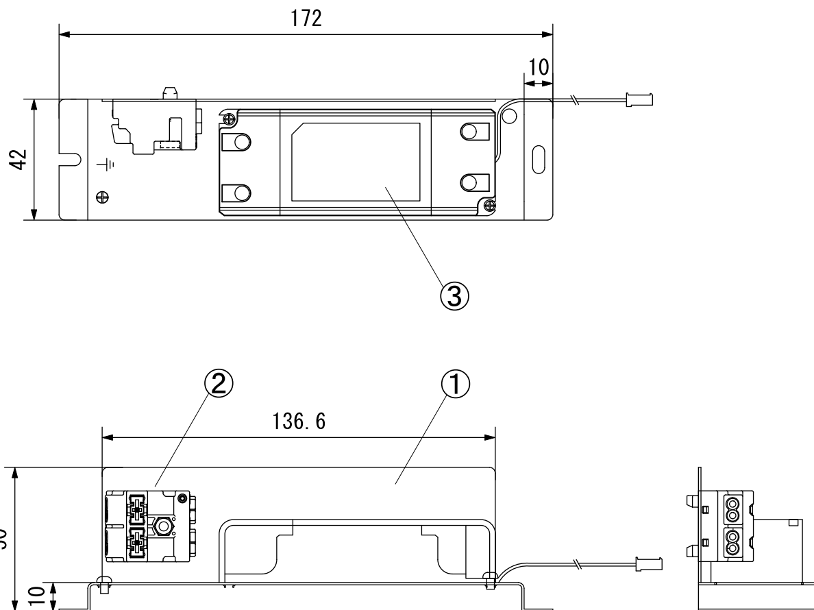
UDL-1164**専用電源ユニット
